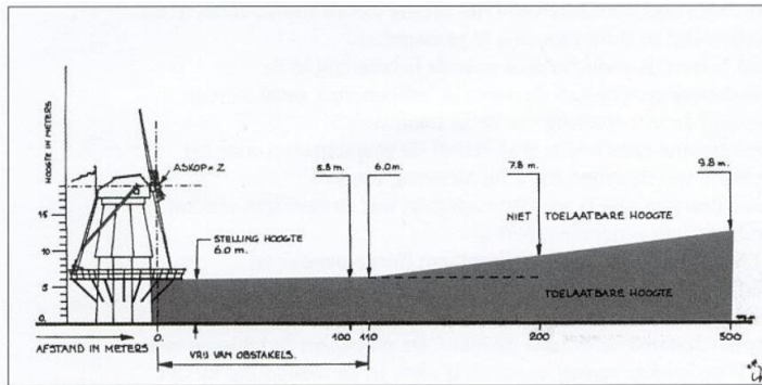
Toelaatbare bebouwingsafstand en -hoogte tot de stellingmolen
